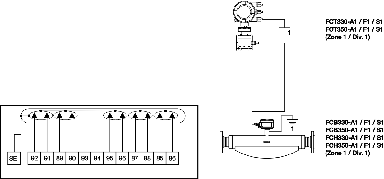
Fig. 30 1 Equipotential bonding (PA)
